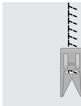
Réglage du point de surjet incliné inversé
