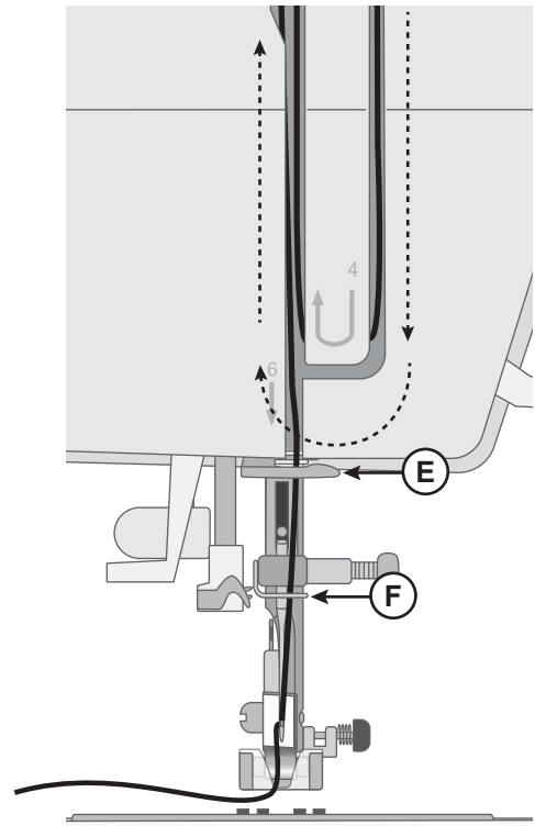
Machine vue de face
